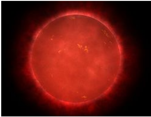
رسم يصور أحد الأقزام الحمر رسمت بريشة فنان
