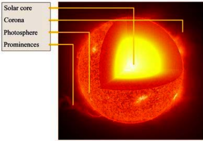
رسم يوضح أقسام الشمس والكرة المضيئة
