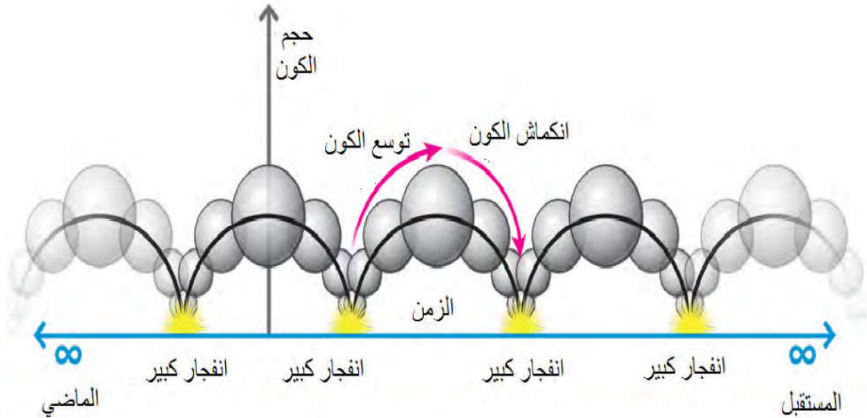
الشكل (١-٣): نموذج الكون المتذبذب - الدوري -.
