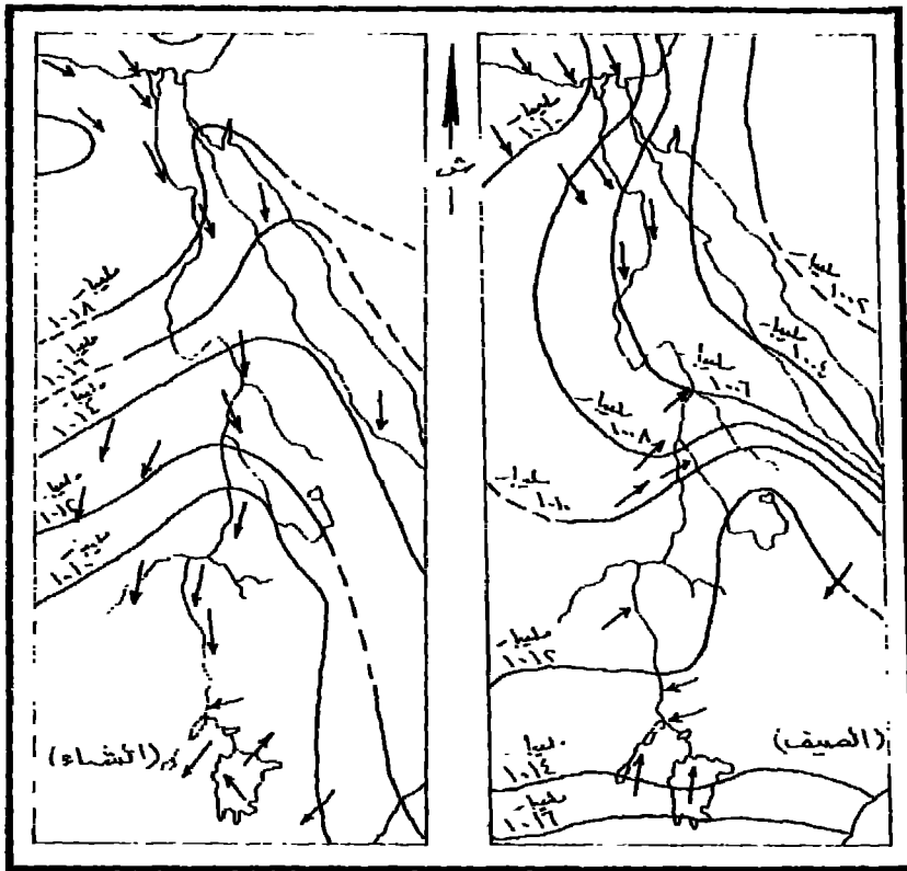
شكل (أ) الضغط الجوي والرياح على حوض النيل في الصيف (يونيو) والشتاء (يناير)
