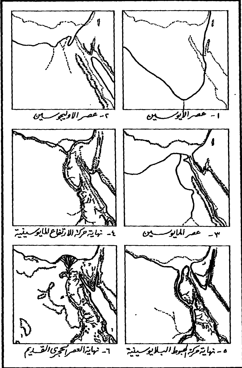
شكل (٢) - توزيع اليابس والماء في مصر في الزمن الجيولوجي الثالث المصدر: موصفي الريه وآخرونه (١٩٥٧م) دلهات في جغرافية مصر ص ١٠٤
