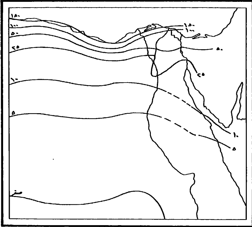
شكل (٩) المتوسط السنوي للهطول بالملي متر
