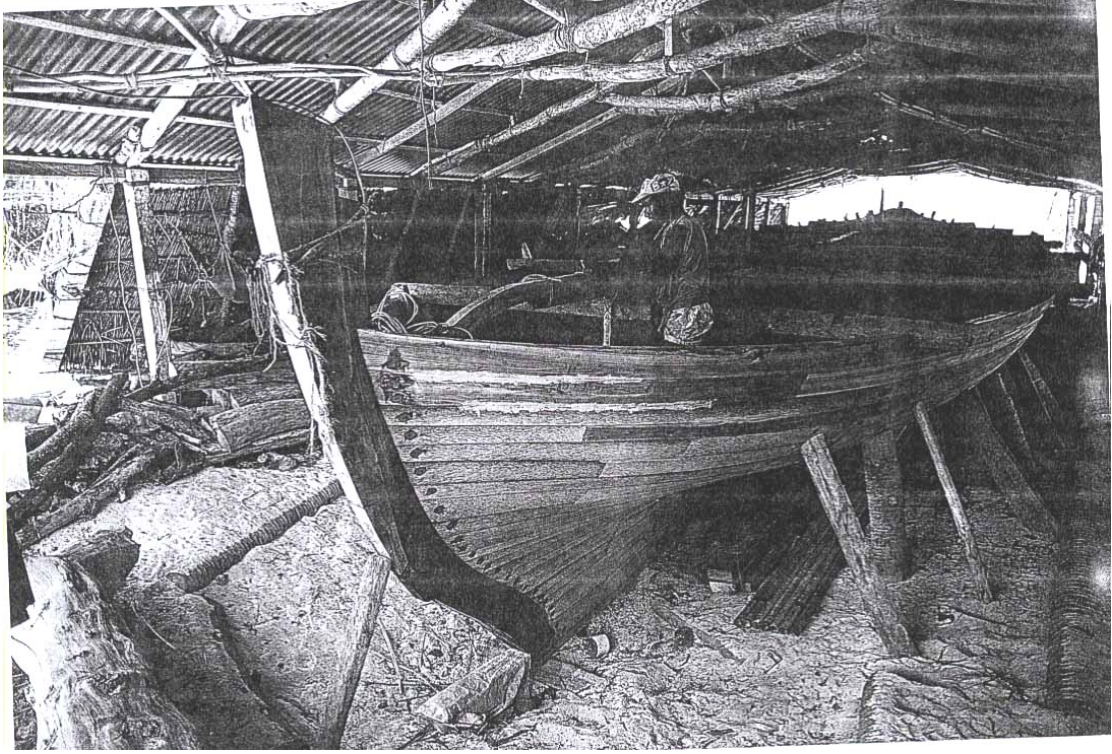
صورة لأحد التجارين المالديفيين يقوم بصناعة المركب دوانى Dhoani في ورشة معدة لذلك بالقرب من البحر (1)
