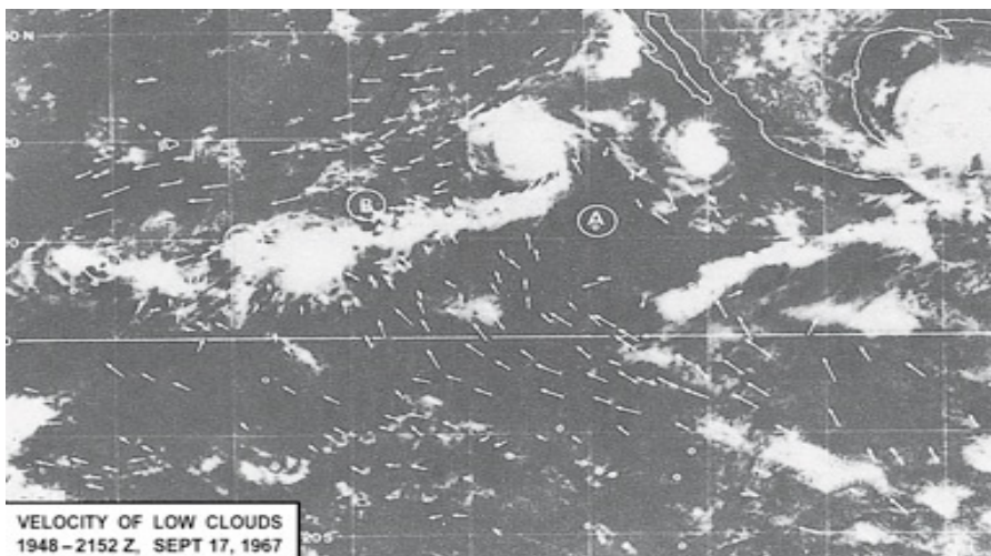
Εικόνα 17: Εικόνα από δορυφόρο που δείχνει τα σύννεφα να κινούνται προς τις περιοχές σύγκλισης B, C, και D. Τα βέλη
