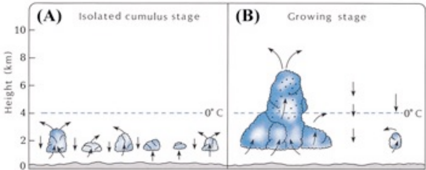
Εικόνα 19: (Α) Απομονωμένα μικρά τμήματα σύννεφων (σωρειτών). (Β) Όταν τα μικρά σύννεφα ενώνονται, τα ανοδικά ρεύματα μέσα στα μεγαλύτερα σύννεφα αυξάνονται, κι έτσι το σύννεφο συσσωρεύεται. Οι σταγόνες νερού απεικονίζονται με •. [ The Atmosphere (Η Ατμόσφαιρα), Anthes και άλλοι, σελ. 269.]
