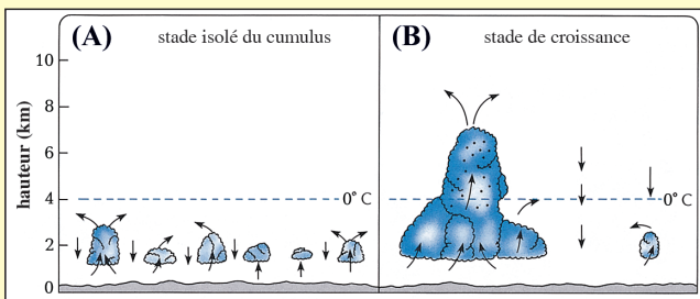
Illustration 19: (A) Fragments de nuages isolés (cumulus). (B) Lorsque les fragments de nuages se rassemblent, les courants d'air ascendants augmentent à l'intérieur du gros nuage nouvellement formé; le nuage se développe alors en hauteur. Les gouttes d'eau sont indiquées par les •. ( The Atmosphere [L'atmosphère], Anthes et al., p. 269.)
