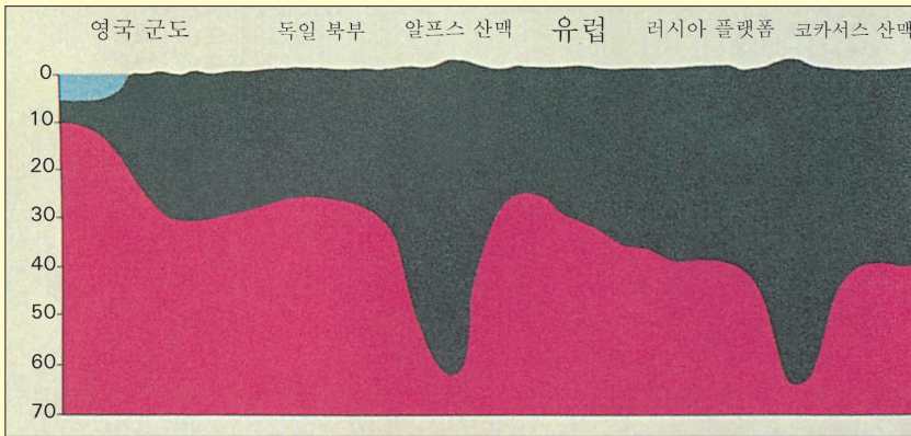
삽화 8: 모형도. 산은 땅 속에 기둥과 같은 깊은 뿌리를 가지고 있다.(Anatomy of the Earth, [지구 해부] Cailleux, p.220)
