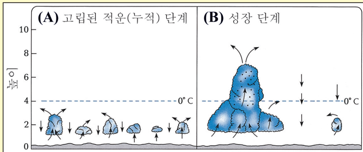
삽화 19: (A) 고립된 작은 적운 조각들. (B) 작은 적운들이 결합하여 만들어진 큰 구름 안에 상승기류가 발생한다. 따라서 구름은 점점 위로 쌓여 올라간다. 물방울은 r 로 표시한다. (The Atmosphere, [대기] Anthes and others, p.269)
