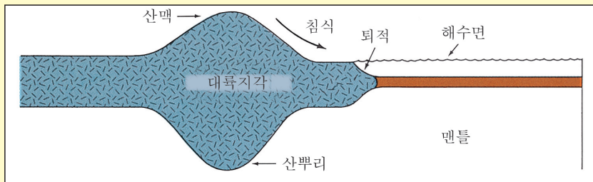
삽화 9: 산 아래의 깊은 뿌리 때문에 마치 기둥을 박아 놓은 것처럼 보인다.(Earth Science, [지구 과학] Tarbuck and Lutgens, p.158)
